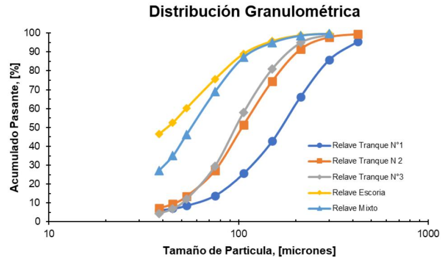
Figura 5-1: Distribución granulométrica muestras relaves ENAMI
